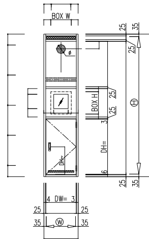
外観図
