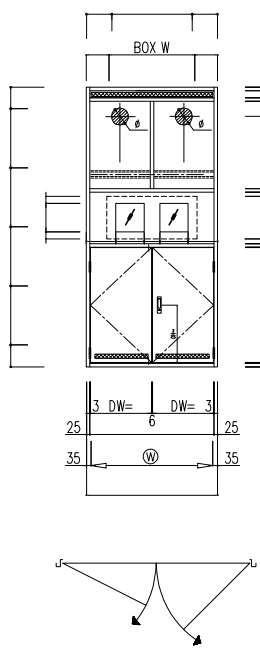
外観図
